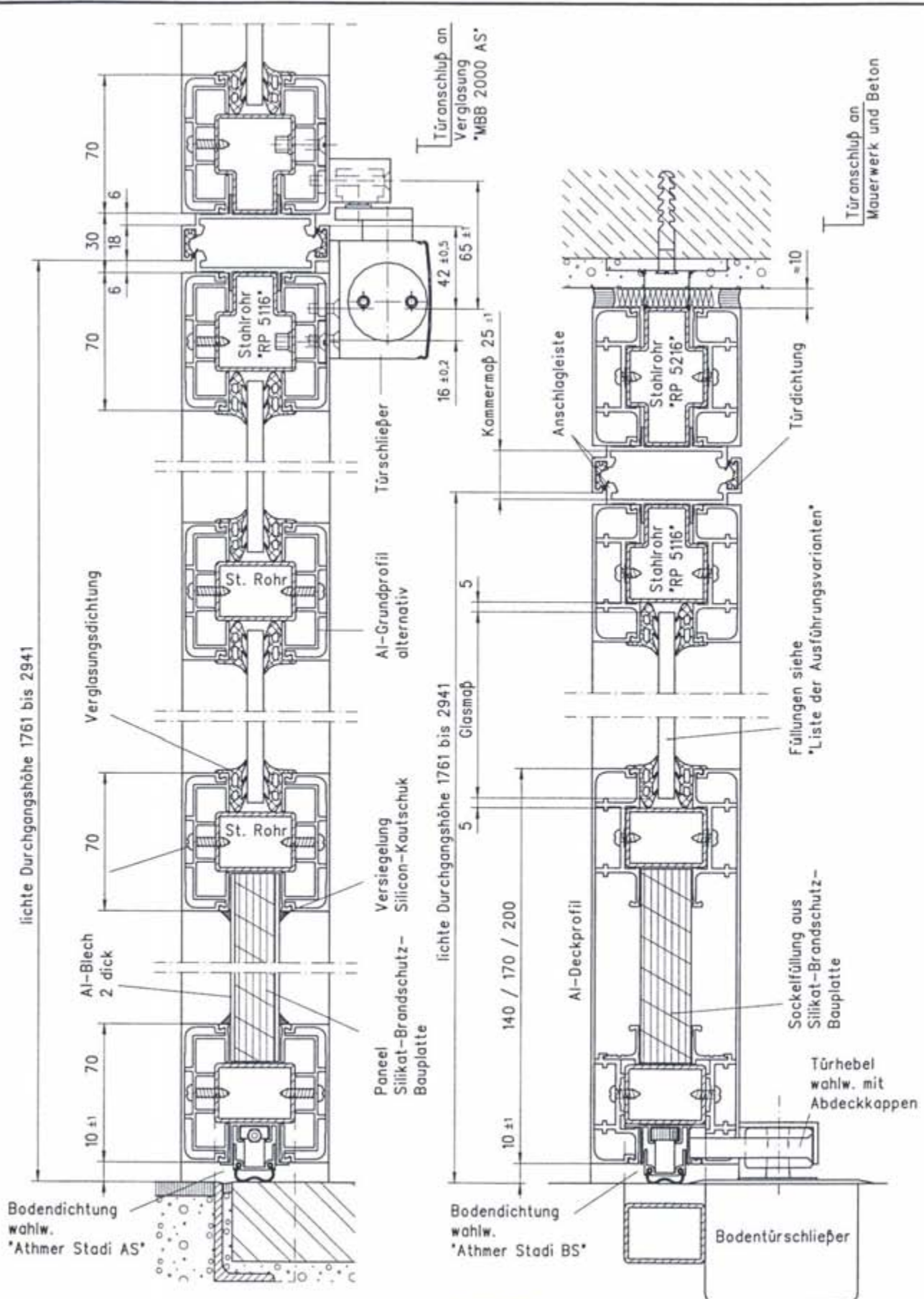
RS-1-Tür *MBB 2000* Vertikalschnitte
