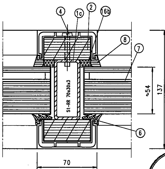
Detail Mittelpfosten -Isolierglasscheibe
