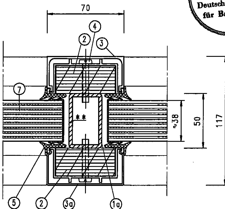
Detail Mittelpfosten -Verbundglasscheibe
